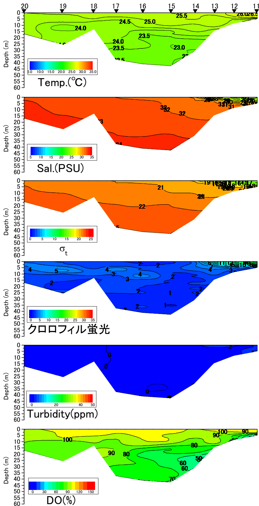
八代海中央ラインの水温(°C)、塩分、密度( \sigma_t )、クロロフィル蛍光強度、濁度、溶存酸素飽和度(DO%)の鉛直面図(国土交通省の調査による) (2014年8月6日)
