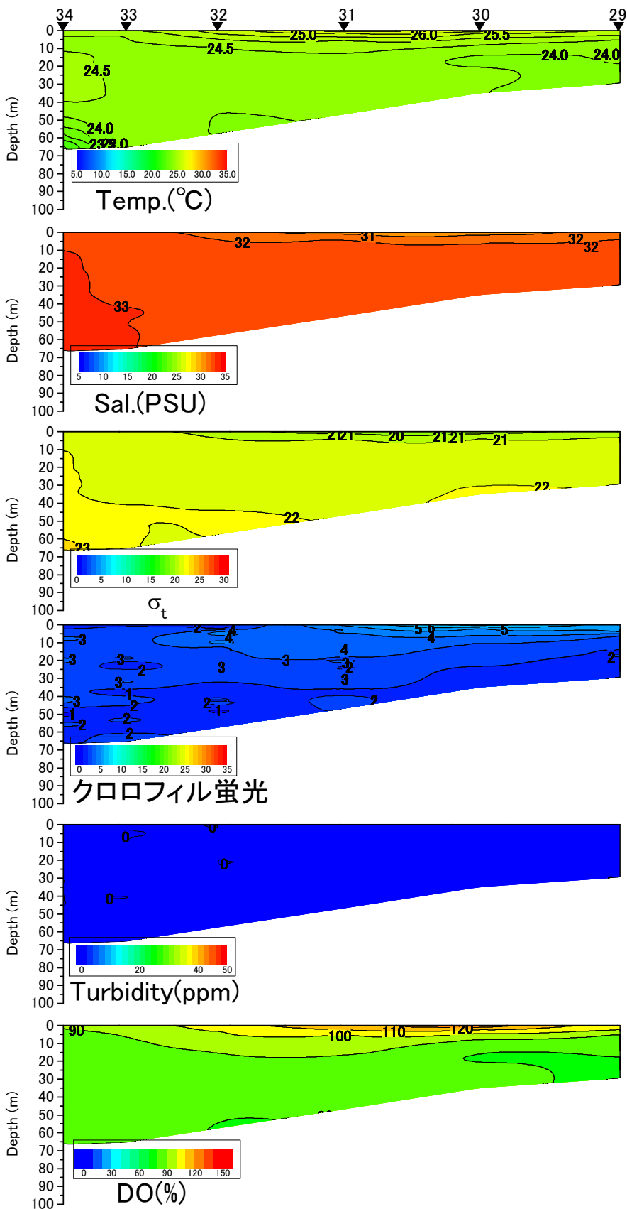
八代海西ラインの水温(°C)、塩分、密度( \sigma_t )、クロロフィル蛍光強度、濁度、溶存酸素飽和度(DO%)の鉛直面図(国土交通省の調査による) (2014年8月6日)
